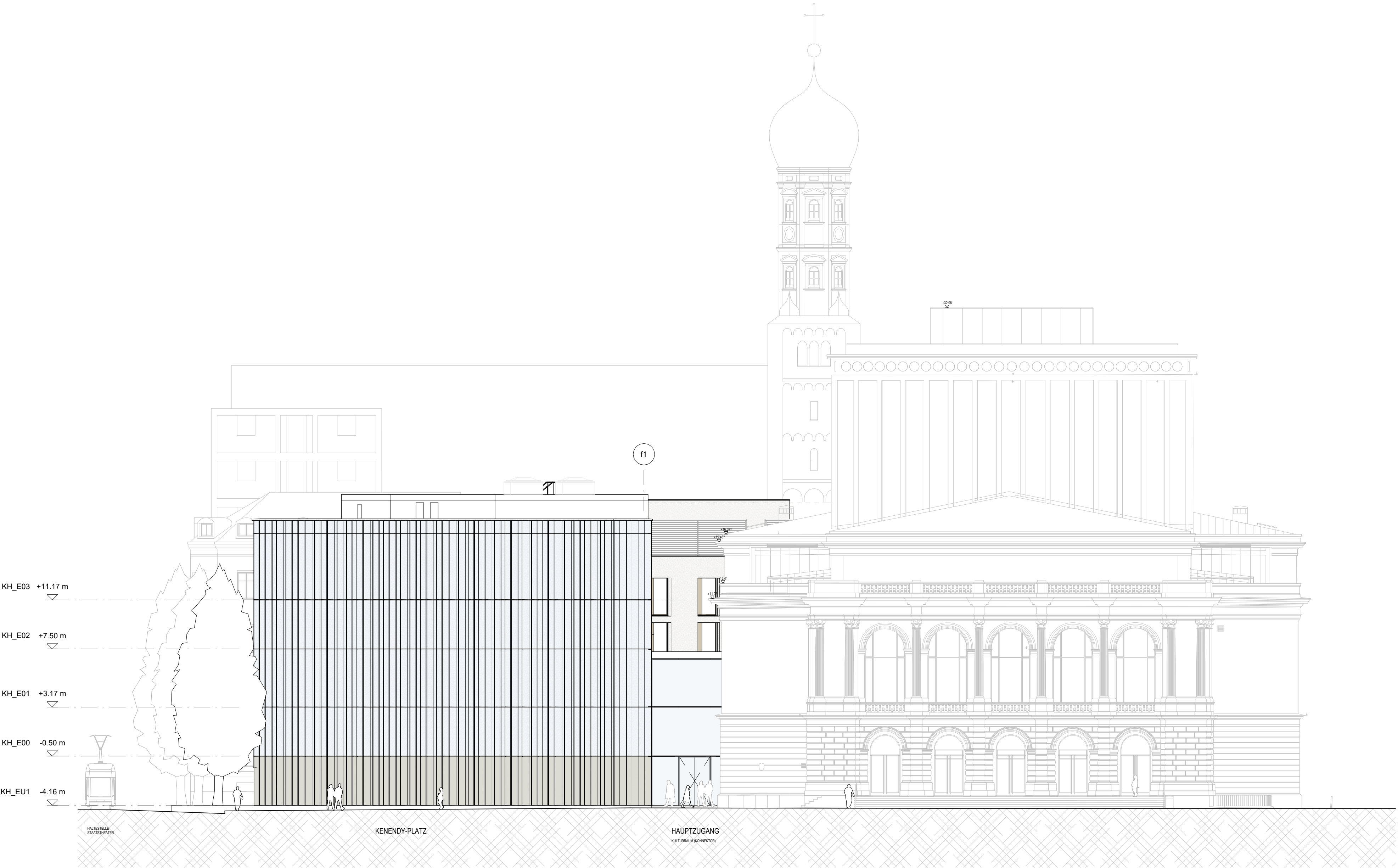
Ansicht 05 - Süd (Kennedy-Platz) 1 : 200
