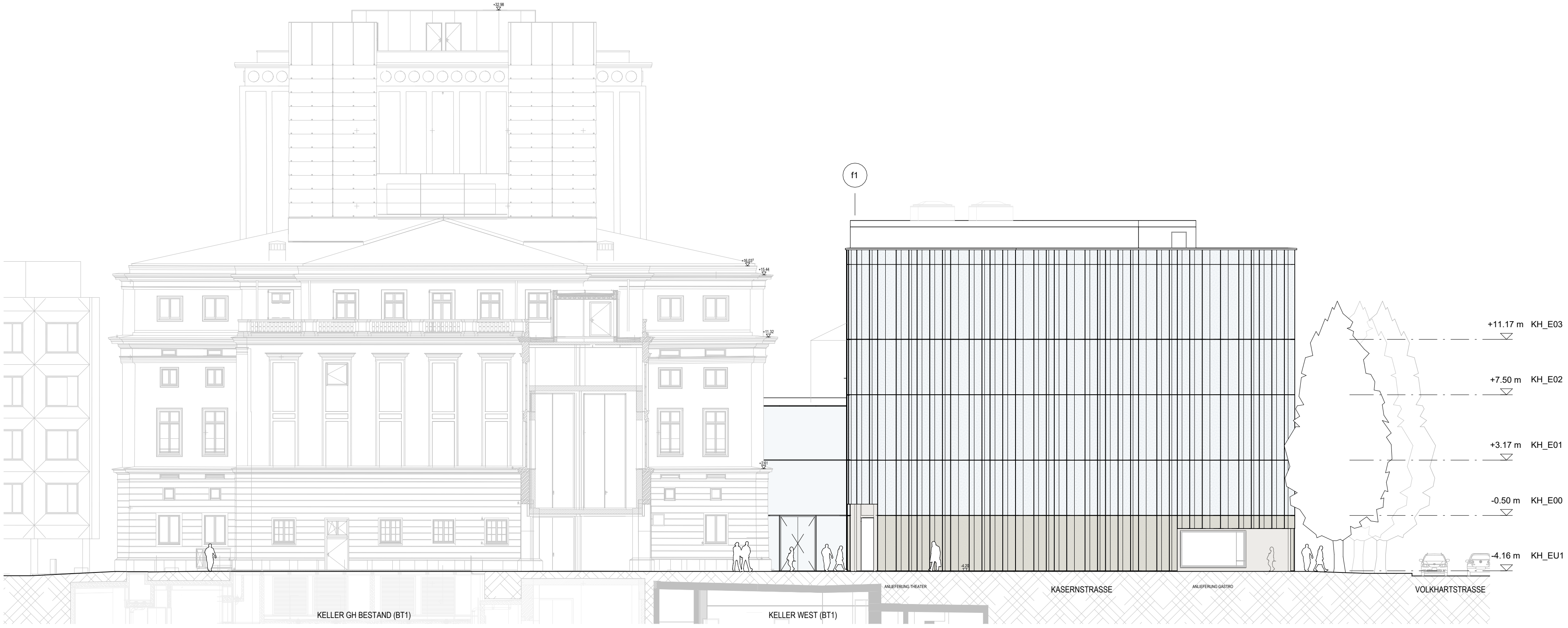
Ansicht 06 - Nord (Kasernstraße) 1 : 200
